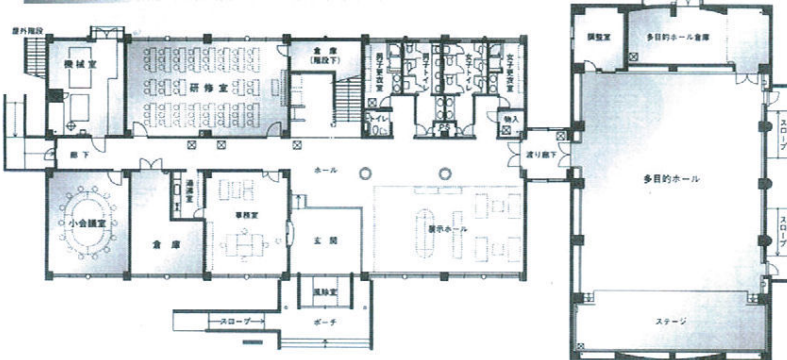
見取図
